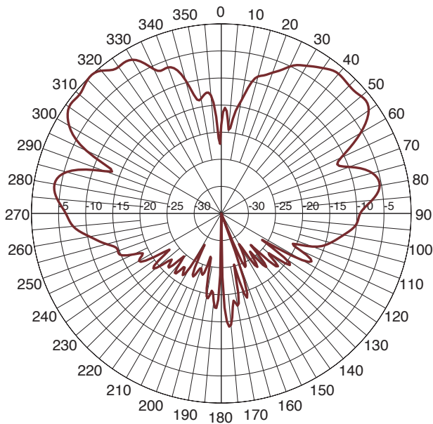
5400MHz - EL PHI90
