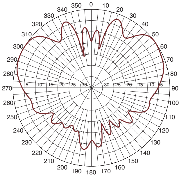
2450MHz - EL PHI90
