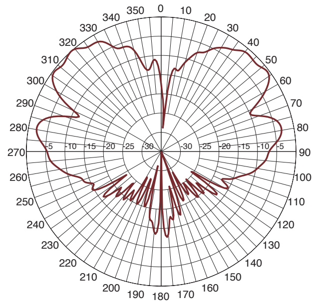
5400MHz - EL PHI0
